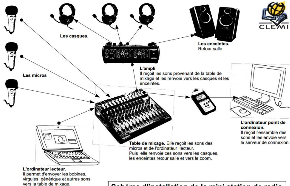
Schéma d'installation de la mini station de radio
